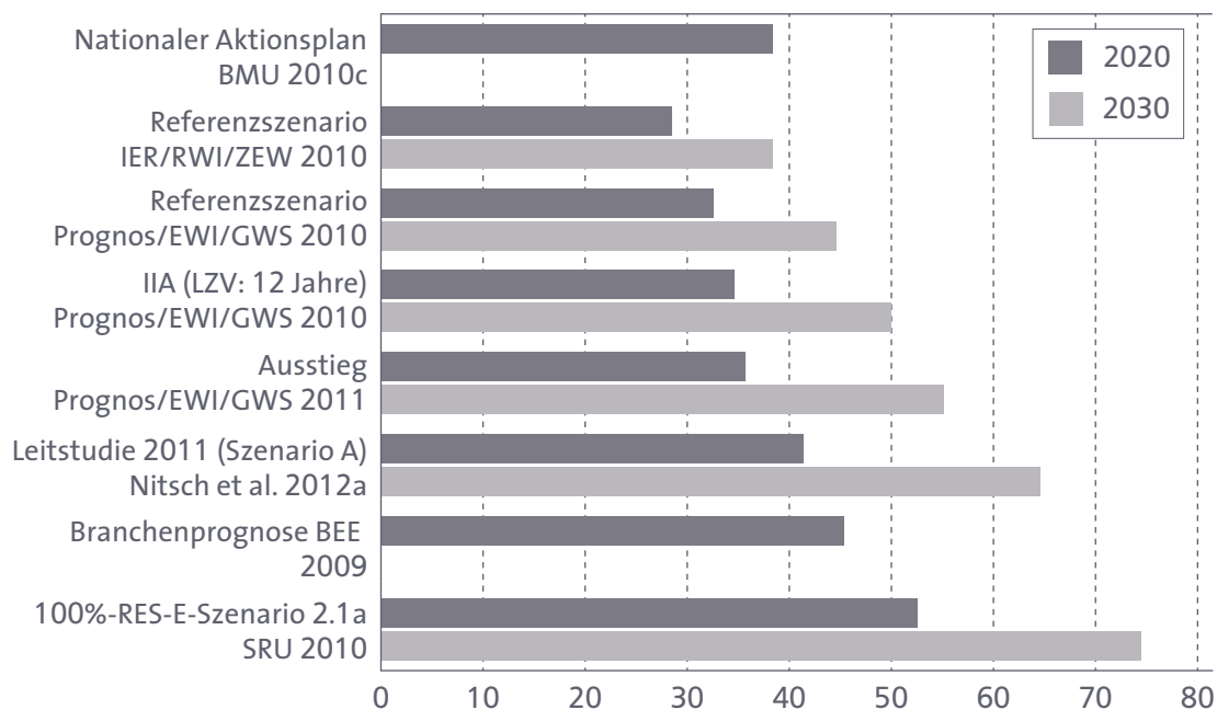
Vergleich von Ausbauszenarien für RES-E (Anteil an der Stromerzeugung in Prozent)
