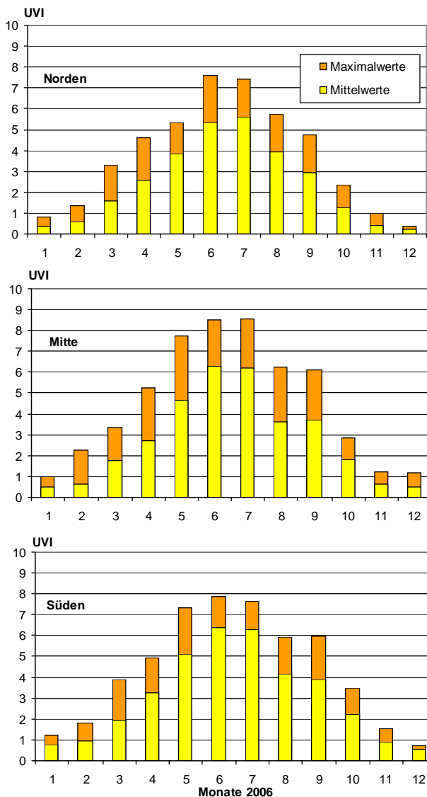
Maximale und mittlere UVI-Werte der Monate im Jahr 2006 im Norden, in der Mitte und im Süden Deutschlands
