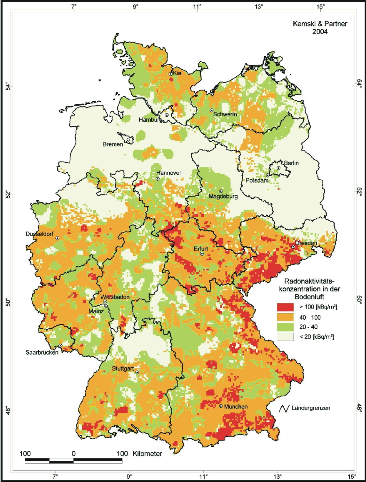
Abbildung I.3-1 Übersichtskarte der Radonkonzentration in der Bodenluft in 1 m Tiefe für die Bundesrepublik Deutschland
